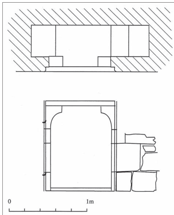
FIG. 1. LA GARDE-ADHÉMAR. ANCIEN CHÂTEAU. Premier étage. Plan et élévation. Relevé Y. Esquieu.
