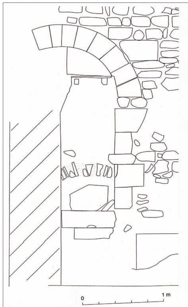
FIG. 5. VIVIERS. 24, rue du Château. Maison élémentaire, premier étage. Relevé Y. Esquieu.
