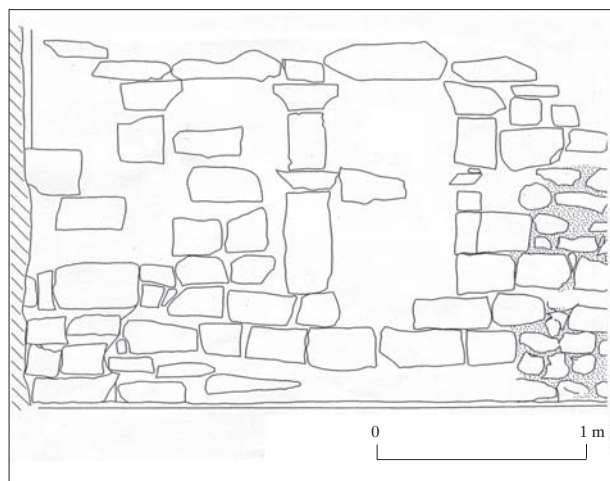
FIG. 4. VIVIERS. Maison rue Montargue. Rez-de-chaussée. Relevé Y. Esquieu.
