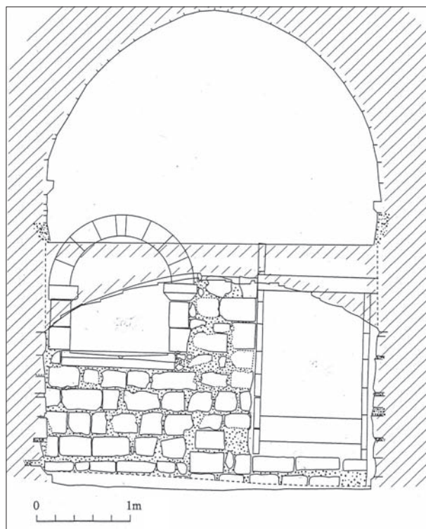
FIG. 2. LA GARDE-ADHÉMAR. RÉSIDENCE ARISTOCRATIQUE. Rez-de-chaussée. L'armoire est coupée par un sol plus tardif. Relevé Y. Esquieu et A. Hartmann-Virnich (dir.).
