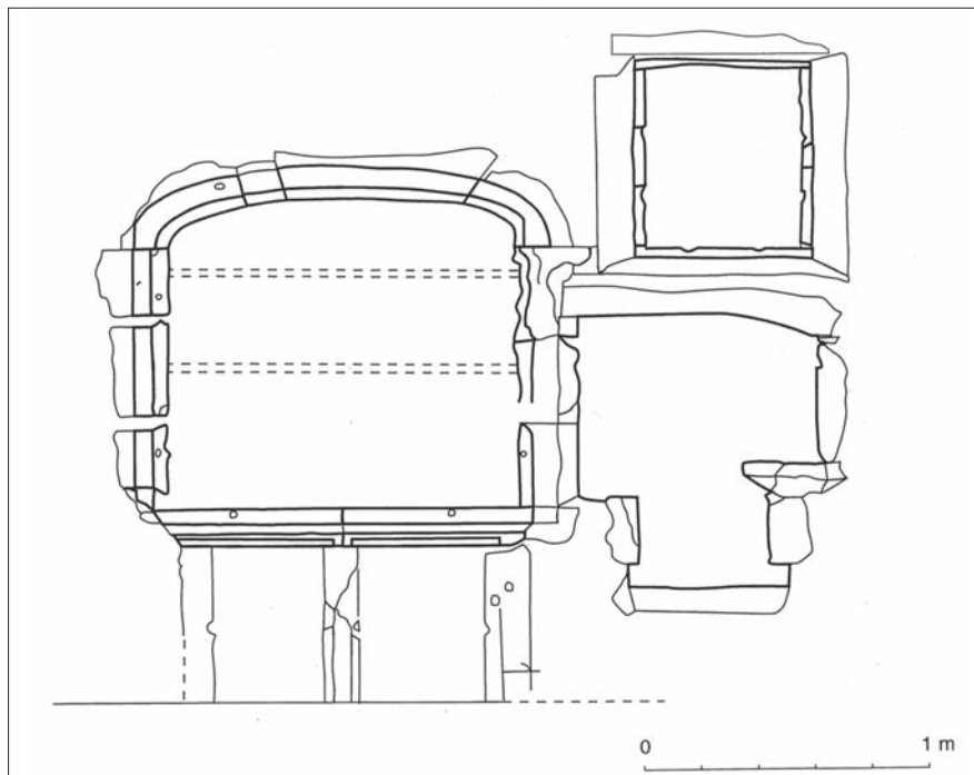
FIG. 12. ROCHEMAURE. PARCELLE 332. Armarium et évier. Relevé Y. Esquieu.
